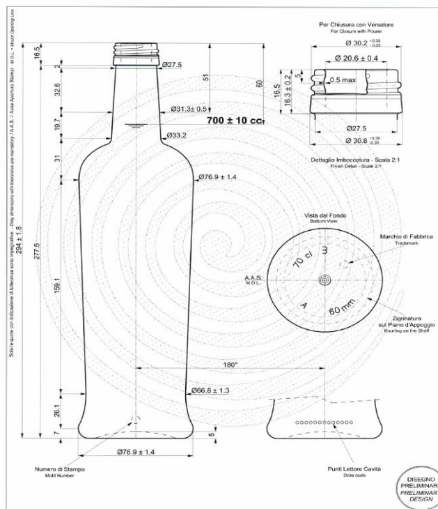
Bottle Design/Disegno della bottiglia
